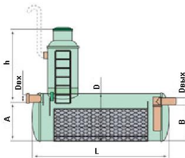
Схема Маслобензоотделителя.
